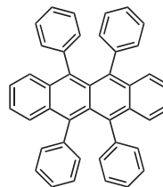
Rubrene
