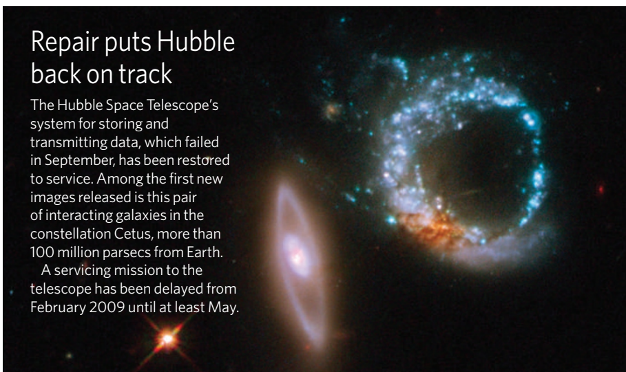
NASA/ESA/AM. LIVIO/STSC
