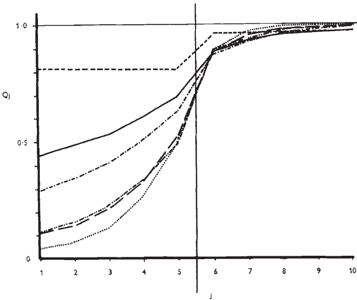
(d) s_1 = s_2 = 0.25; \quad t_1 = 1, \quad t_2 = 5
